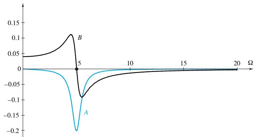
Figura 4.5 Amplitudes de vibración en torno a una resonancia
