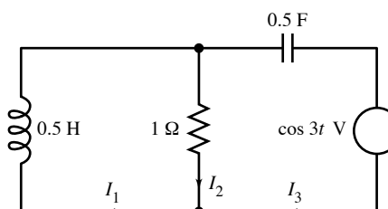
Figura 5.36 Red RLC para el problema 13
