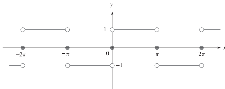
Figura 10.7 La función límite de la serie de Fourier para f(x) = \begin{cases} -1, & -\pi < x < 0, \\ 1, & 0 < x < \pi \end{cases}
