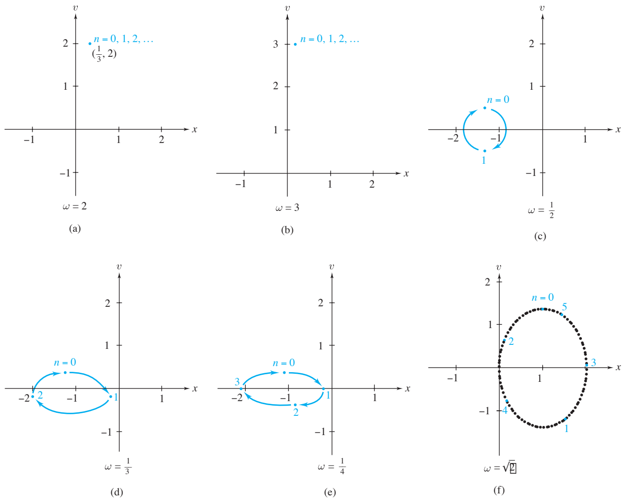
Figura 5.37 Secciones de Poincaré para la ecuación (1) para diversos valores de \omega
