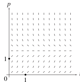
Figura B.4 Campo de direcciones para el problema 5(a)
