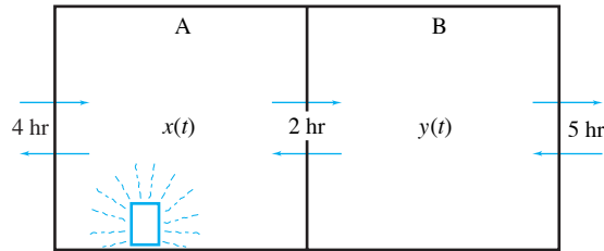
Figura 5.5 Edificio con dos zonas, una de ellas calentada
