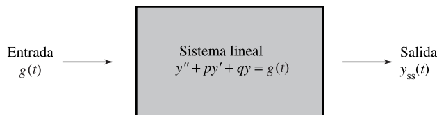
Figura 7.30 Diagrama de bloque que muestra un sistema lineal
