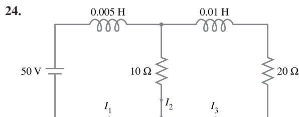
Figura 7.29 Red RL para el problema 24
