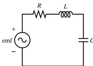
Figura 1.3 Diagrama de un circuito RLC en serie
