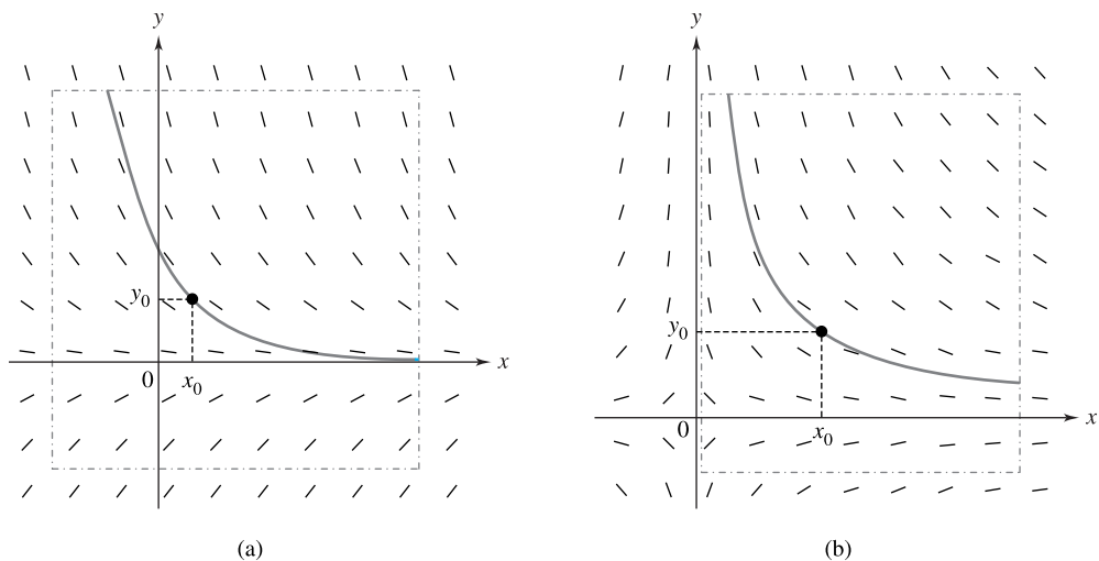
Figura 1.8 (a) Una solución para dy/dx = -2y (b) Una solución para dy/dx = -y/x
