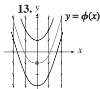
Figura B.7 Solución del problema 11
