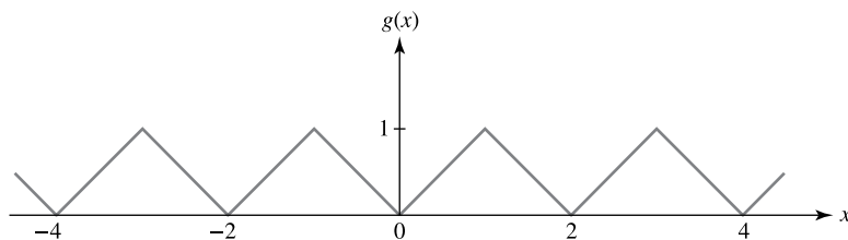
Figura 10.9 Extensión periódica de f(x) = |x| , -1 < x < 1
