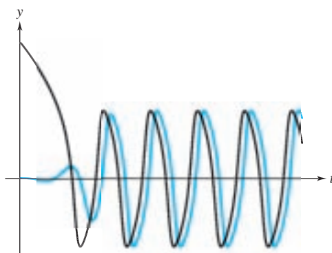
Figura 4.17 Soluciones a la ecuación de van der Pol
