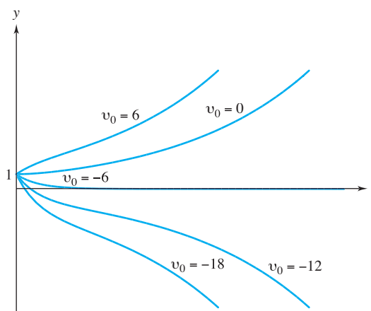
Figura 4.8 Gráficas solución para el ejemplo 4
