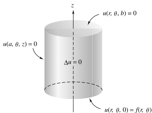
Figura 10.27 Problema de Dirichlet para el cilindro
