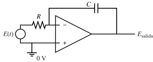
Figura 3.19 Integrador con amplificador operacional
